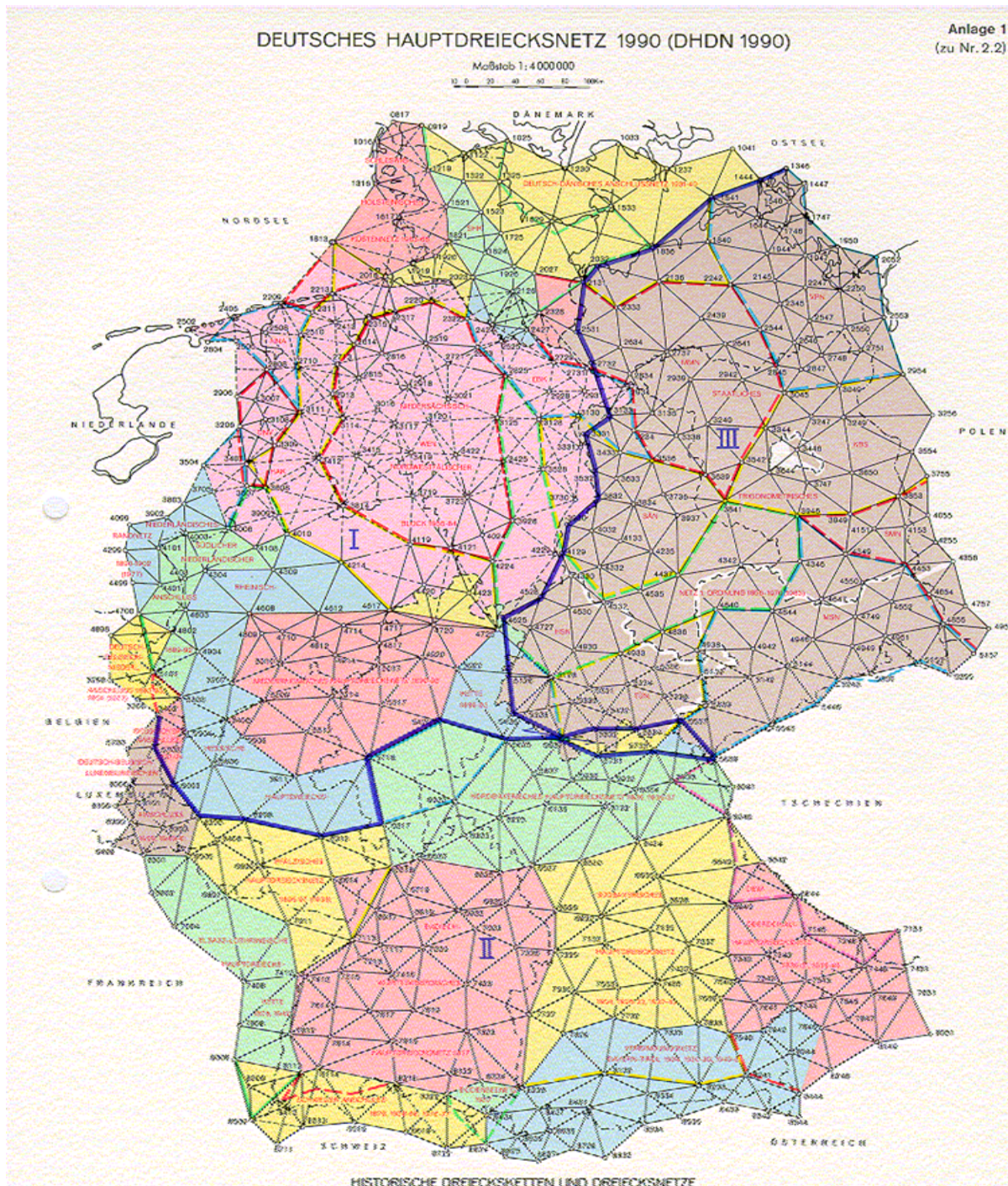
Abbildung 1: Deutsches Hauptdreiecksnetz 1990 mit Netzteilen
