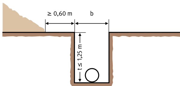
Abb. 19 Maximale Tiefe ohne Verbau und Schutzstreifen
