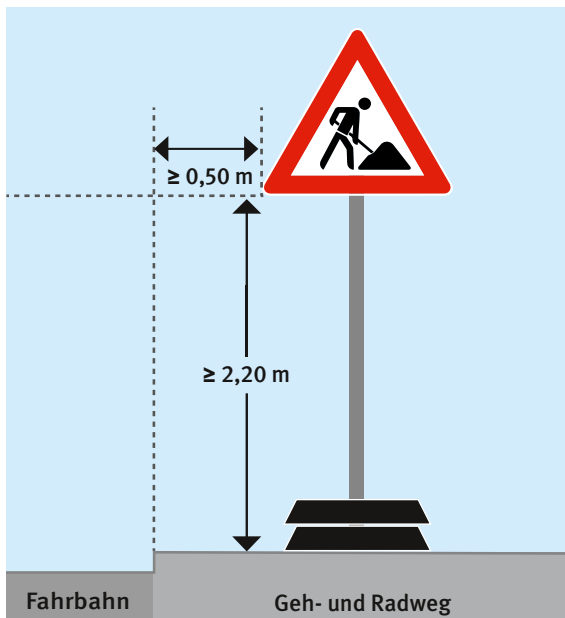
Abb. 15 Regelausführung innerorts
