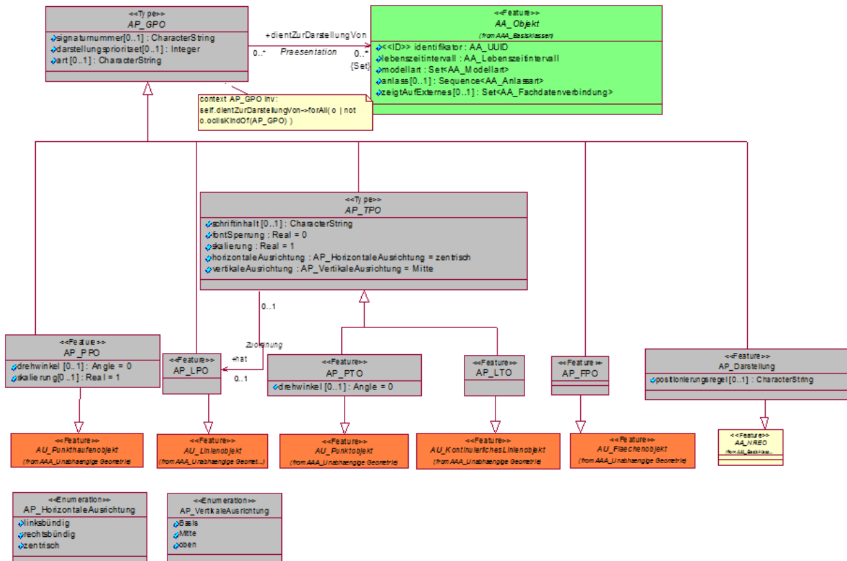
Abbildung 20: AAA-Präsentationsobjekte
