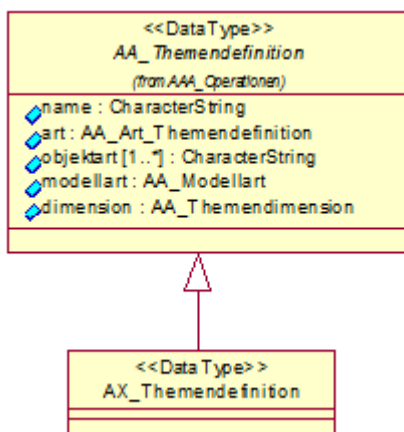
Abbildung 3: Klassendiagramm AX_Themendefinition
